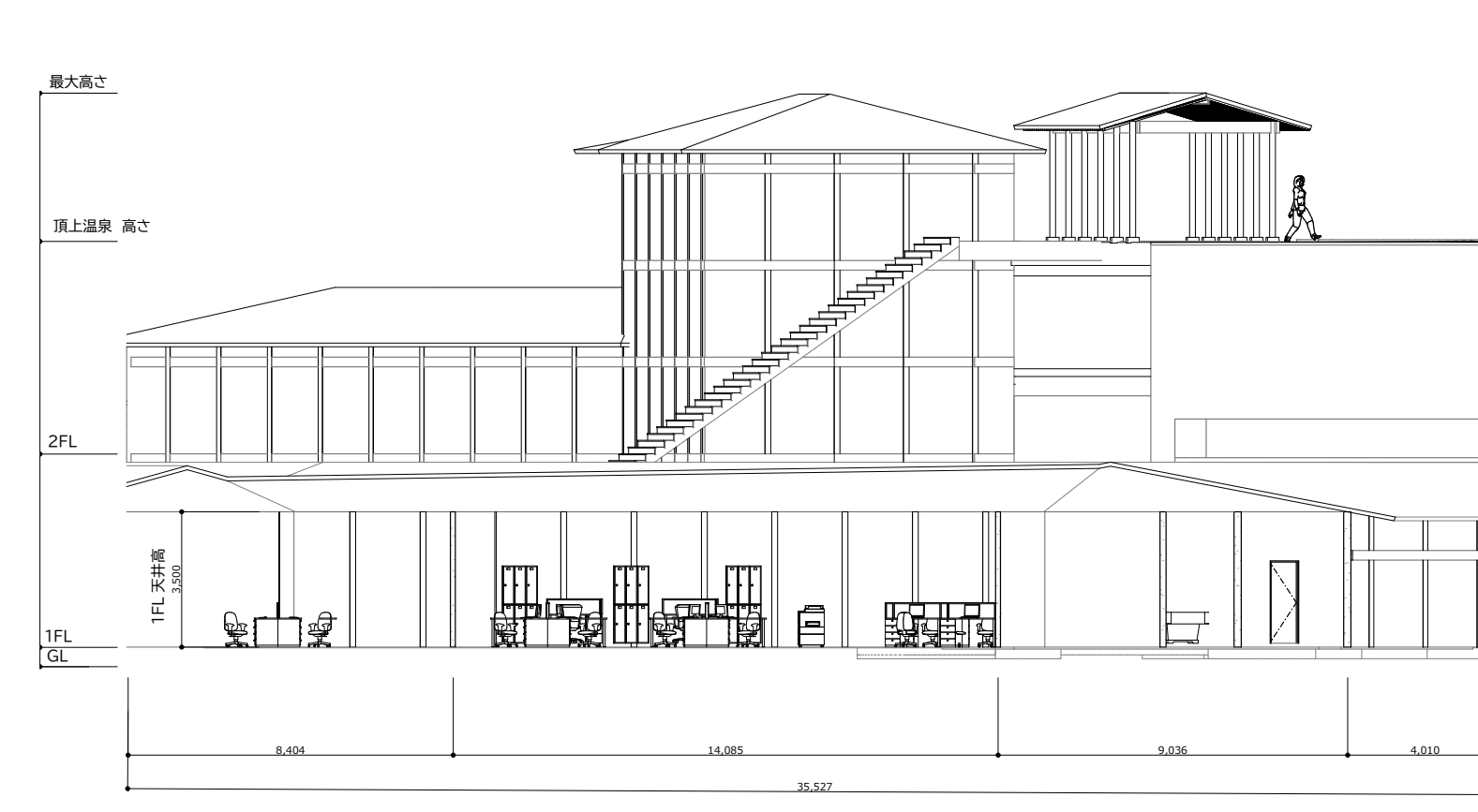
温泉エリア 断面図 1:200
