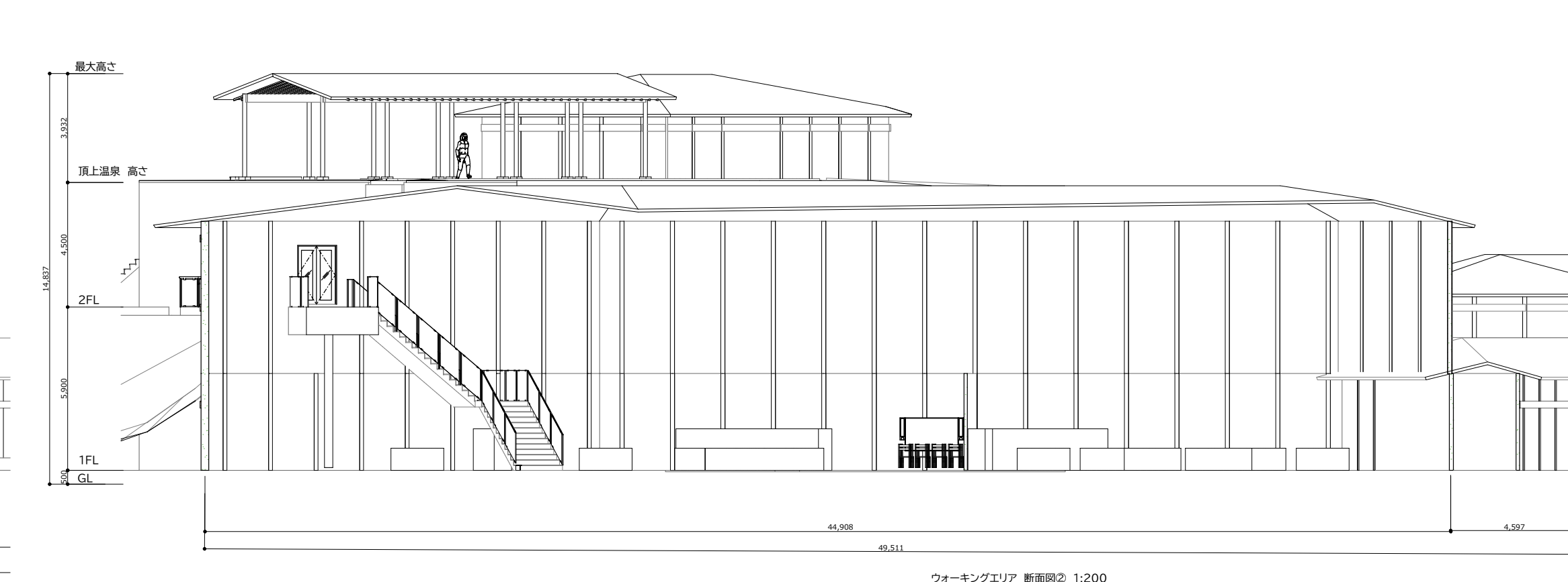
ワーキングエリア 断面図② 1:200
