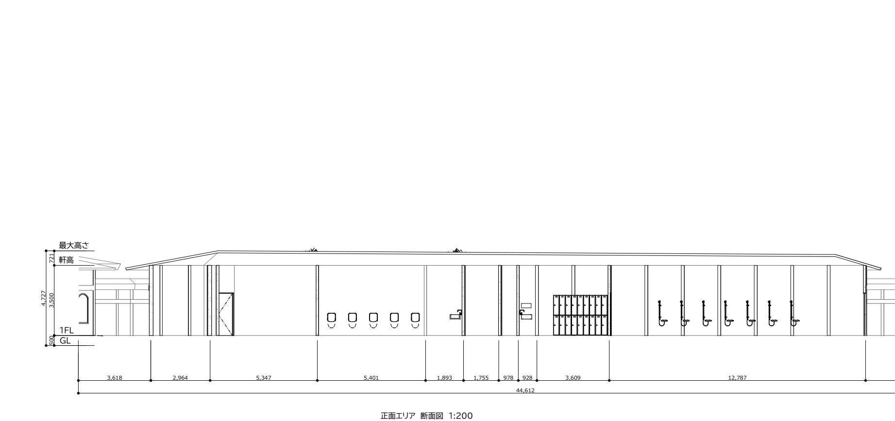
正面エリア 断面図 1:200
