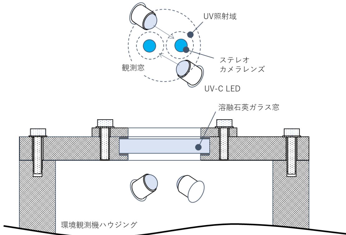
図1 藻類付着防止観測窓の基本構成図
