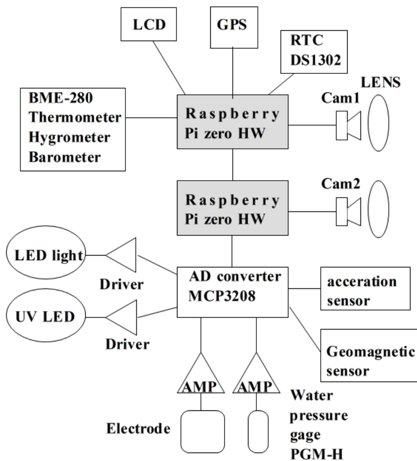
図 2 2 台の Raspberry Pi を用いる構成
