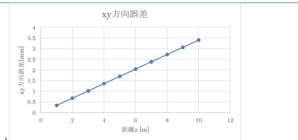
図 1 4 z 方向距離に対する xy 方向の誤差
