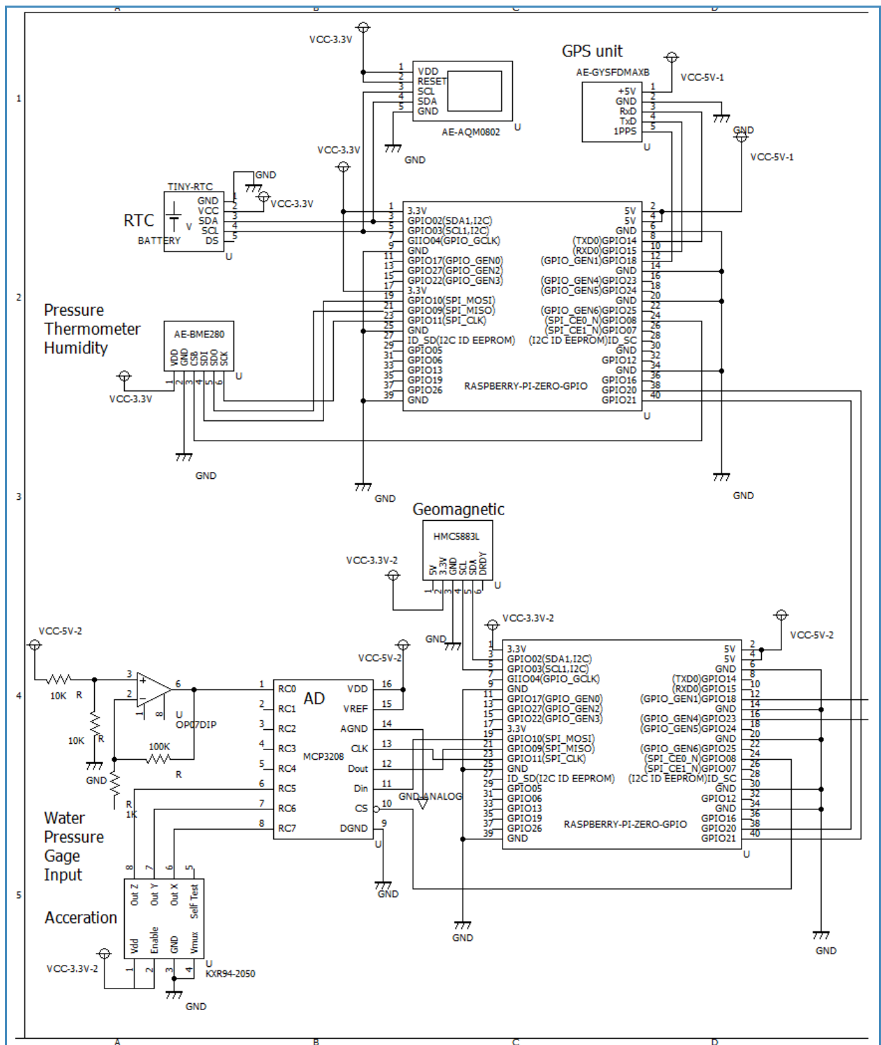
図4 回路構成 (左半分)
